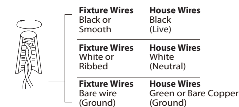
Fig. 2 Wiring
