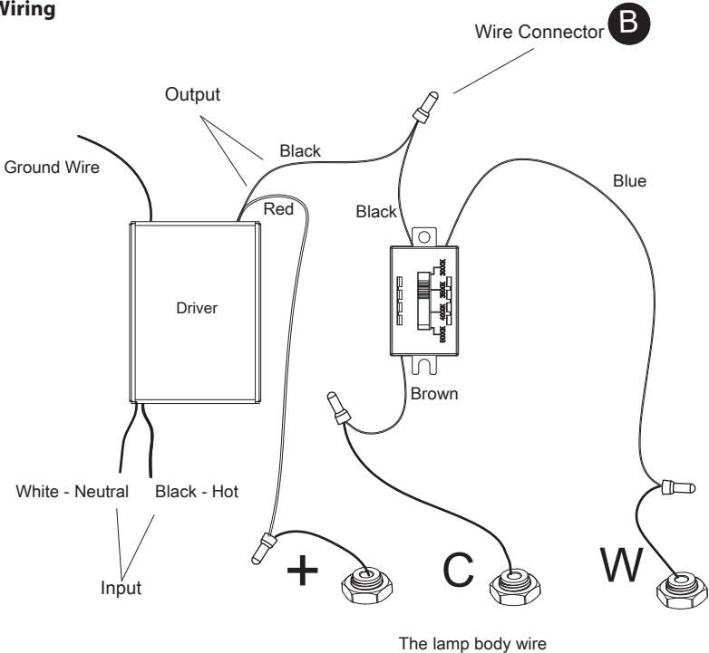
Fig. 4 Wiring
