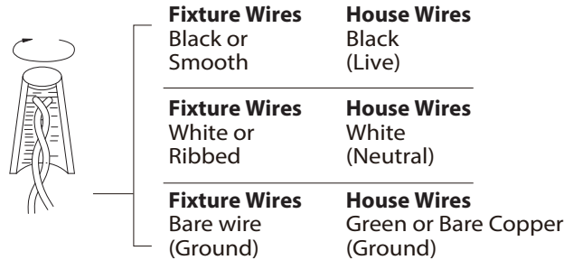
Fig. 2 Wiring
