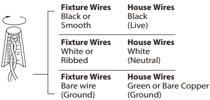
Fig. 2 Wiring
