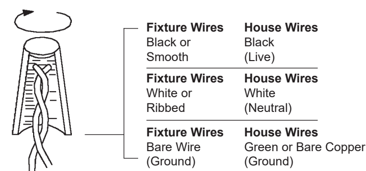
FIG. 3 Wiring
